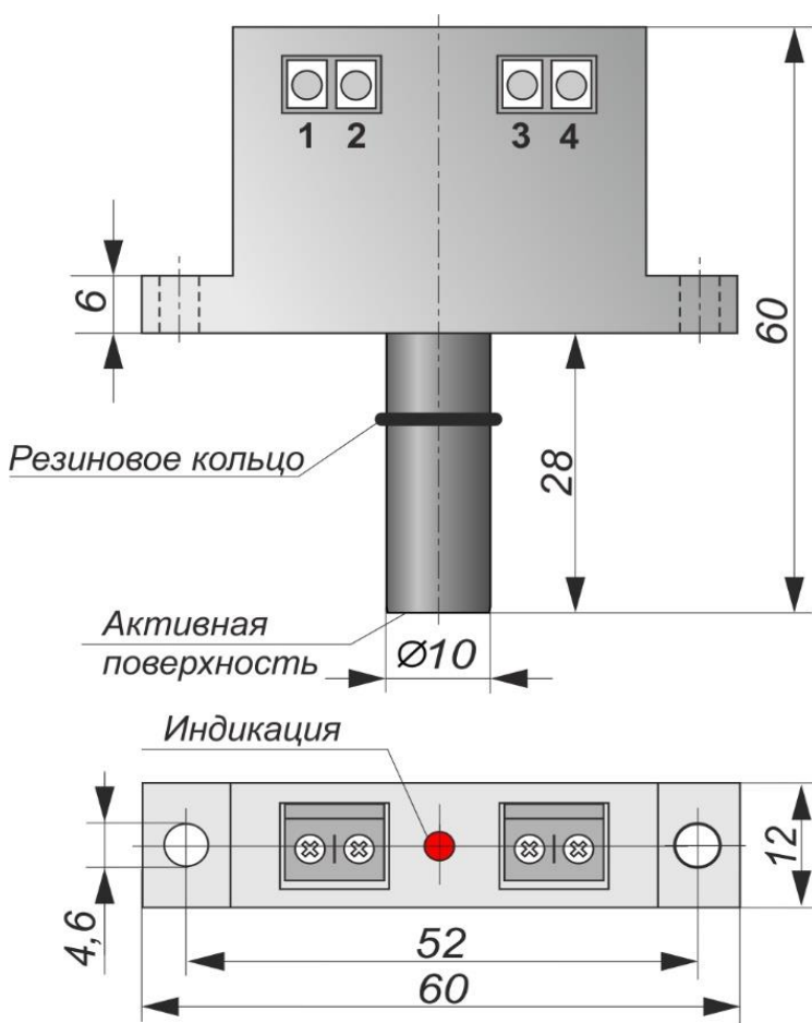
Габаритный чертеж
